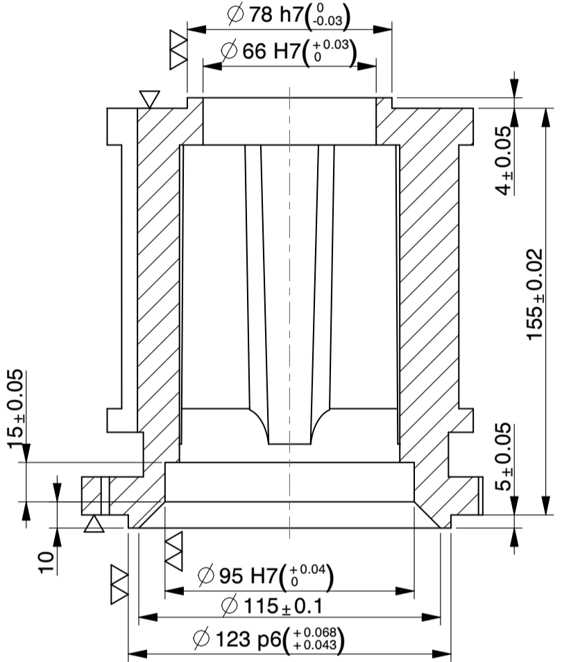
SECTION A-A
